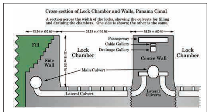
Figura 12 - Uno schema dei cunicoli del bacino.
