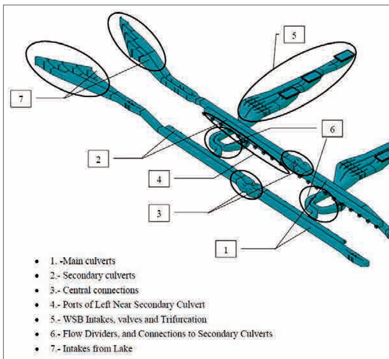
Figura 13 - Sistema di riempimento e vuotamento delle nuove chiuse. Si notino i collegamenti con le vasche di riuso dell'acqua (Water Saving Basin).
