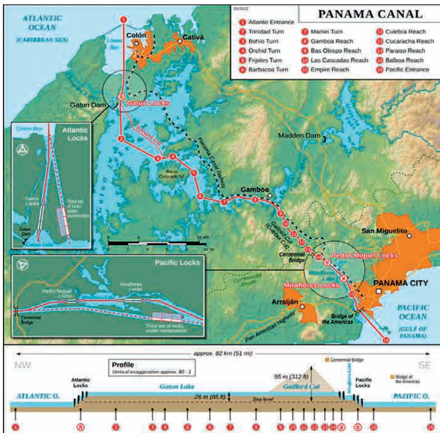
Figura 6 - Pianta e sezione del Canale di Panama.
